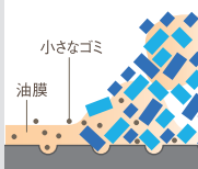
汚れ除去機構 模式図
