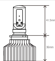
PSX26W(イエロー)
